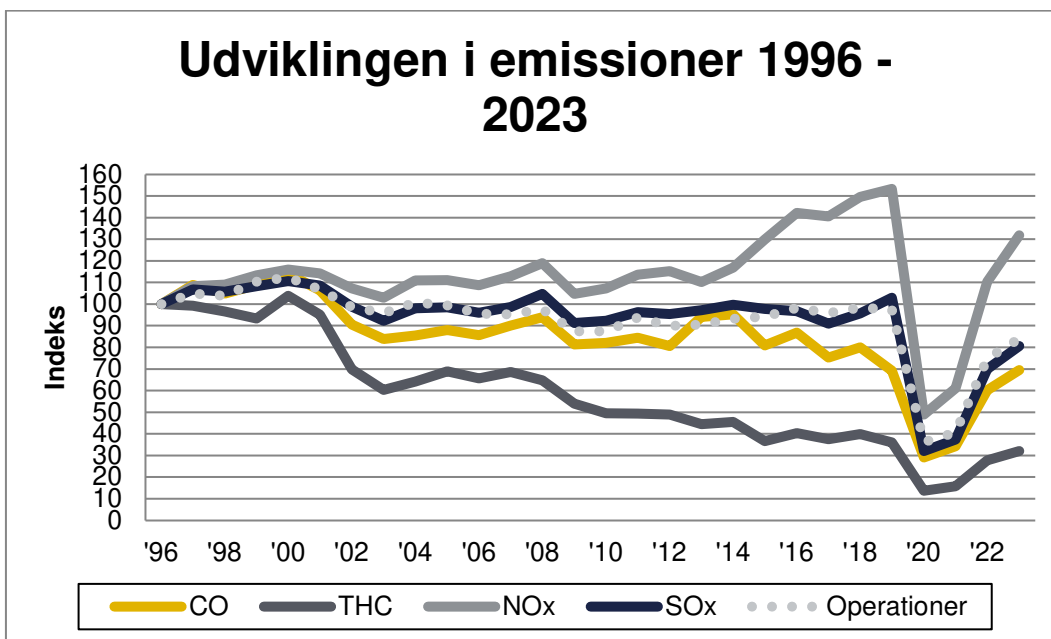
Figur 1: Udviklingen i emissioner fra fly i perioden 1996 – 2023.
