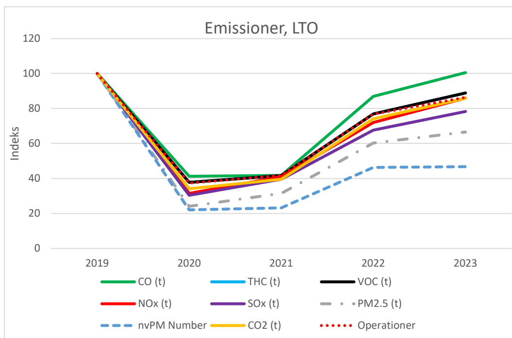
Figur 3: Trafik og emissioner udsendt i hele LTO-cyklen (alle aktiviteter under 3.000 fod)
