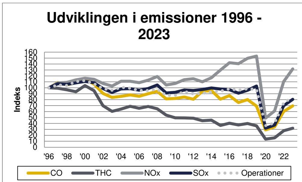
Figur 12. Den beregnede udvikling i emissioner fra flyenes APU og hovedmotorer under gennemførte LTO-cykler i perioden 1996-2023.
