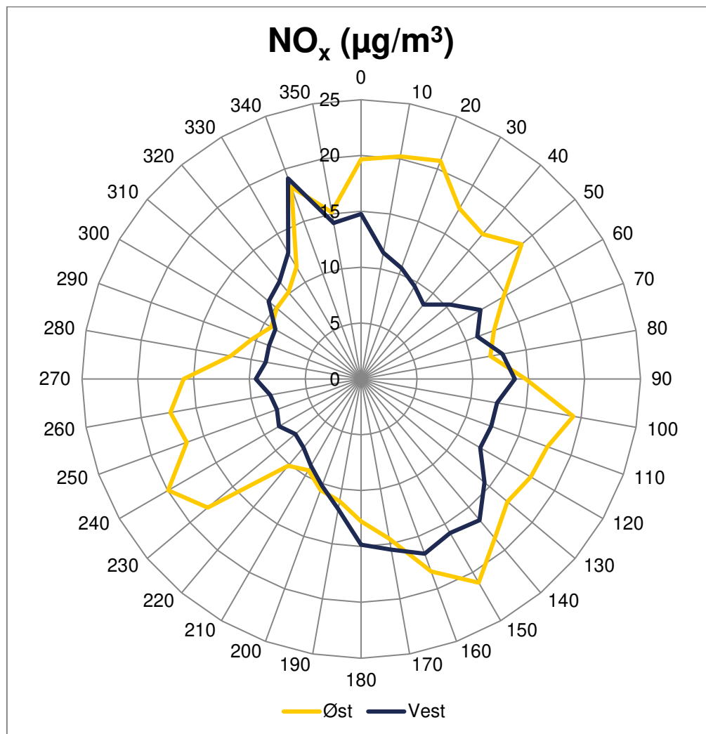
Figur 6. Den gennemsnitlige koncentration af NO x ved forskellige vindretninger i 2023.
