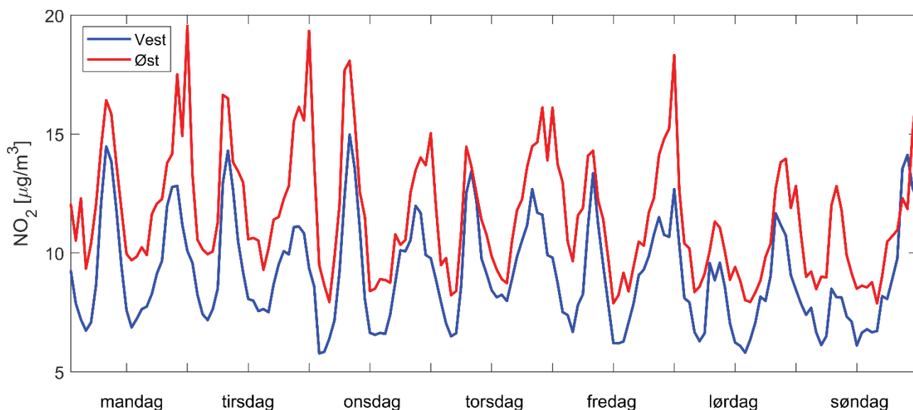
Figur 7. Gennemsnitlig døgnvariation i 2023 af koncentrationen af NO 2 på Station Vest og Øst.
